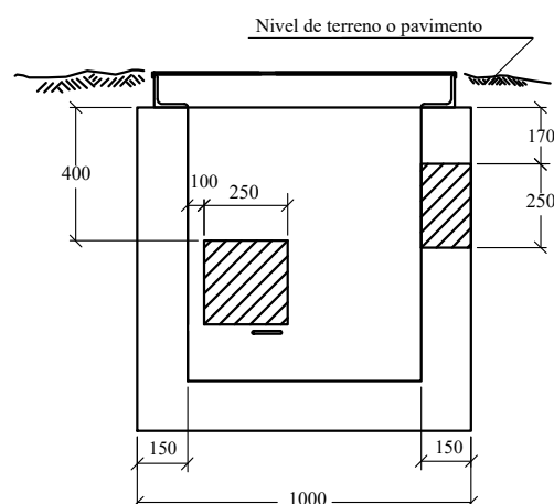
Sección B-B'
